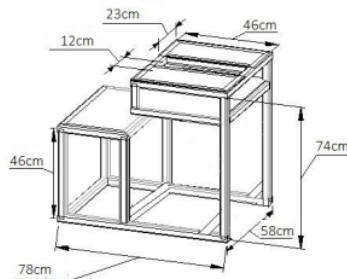
Gambar 1 Rancangan Meja Kursi Porting
