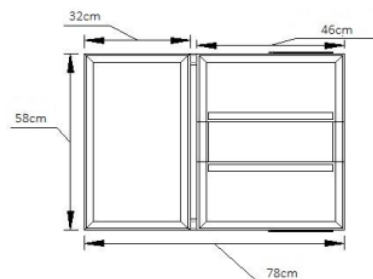
Gambar 3 Tampak Atas
