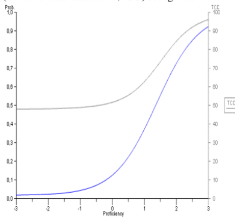
Gambar 9. Kurva Karakteristik Butir 80
