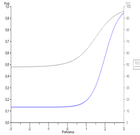
Gambar 8. Kurva Karakteristik Butir 45
