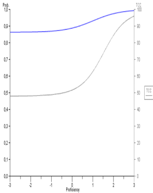
Gambar 6. Kurva Karakteristik Butir 83
