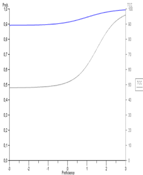
Gambar 7. Kurva Karakteristik Butir 93
