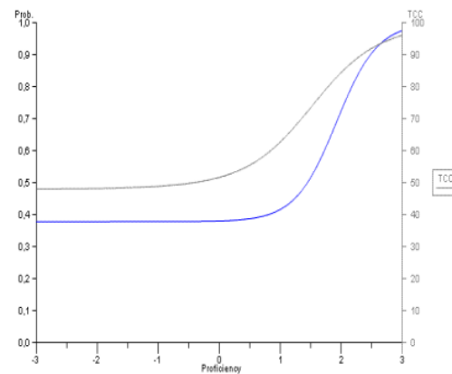
Gambar 5. Kurva Karakteristik Butir 38
