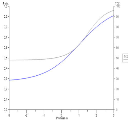
Gambar 4. Kurva Karakteristik Butir 8
