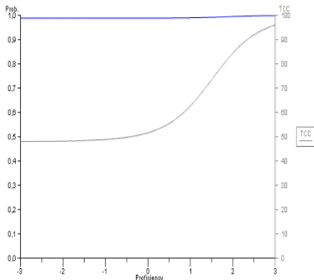
Gambar 10. Kurva Karakteristik Butir 68
